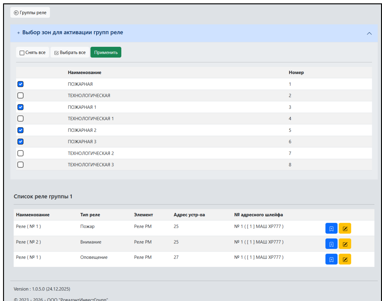
Рис. 55. Скриншот окна меню «Выбор зон для активации групп реле»
