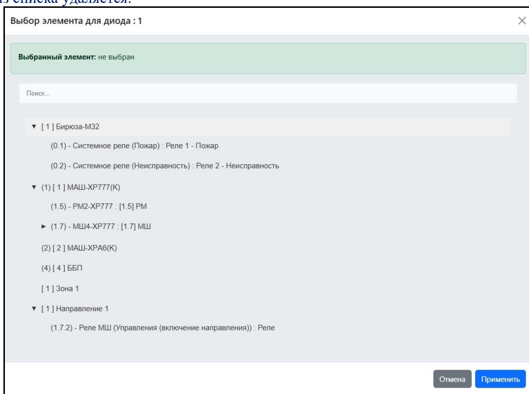
Рис. 40. Скриншот окна со списком элементов для присвоения светодиодам ВПИУ (базовая)
