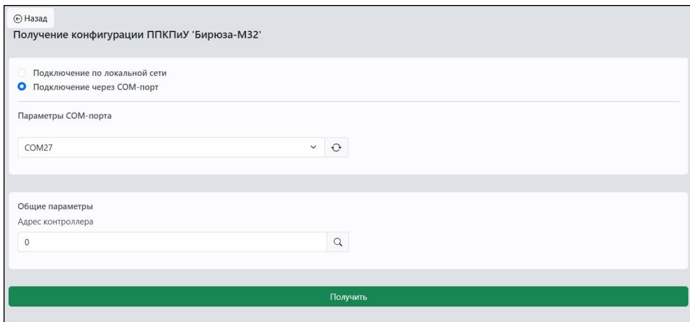
Рис. 66. Скриншот окна вкладки «Получение конфигурации ППКПиУ 'Бирюза-М32'»
