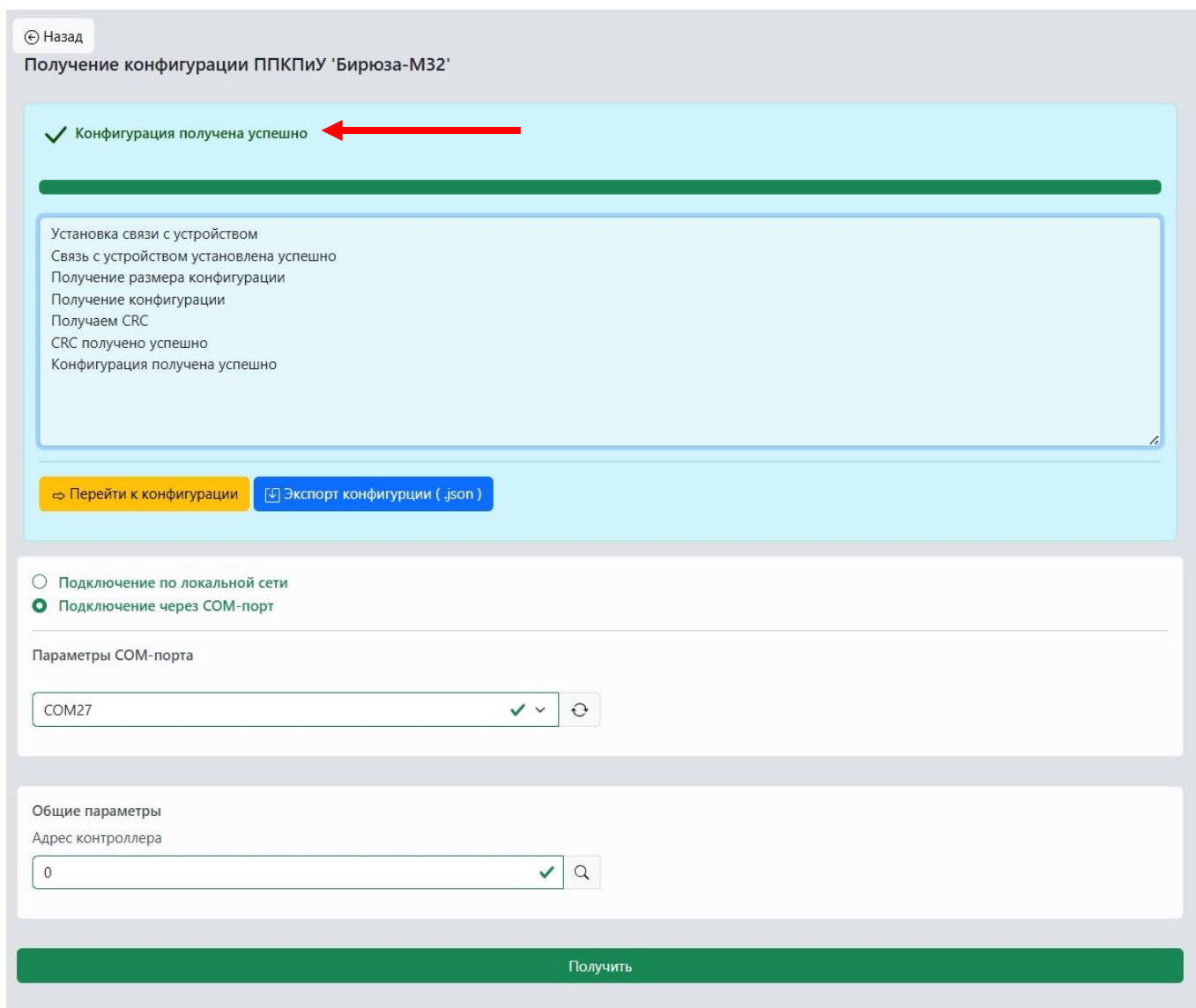
Рис. 67. Скриншот окна получения конфигурации из памяти прибора
