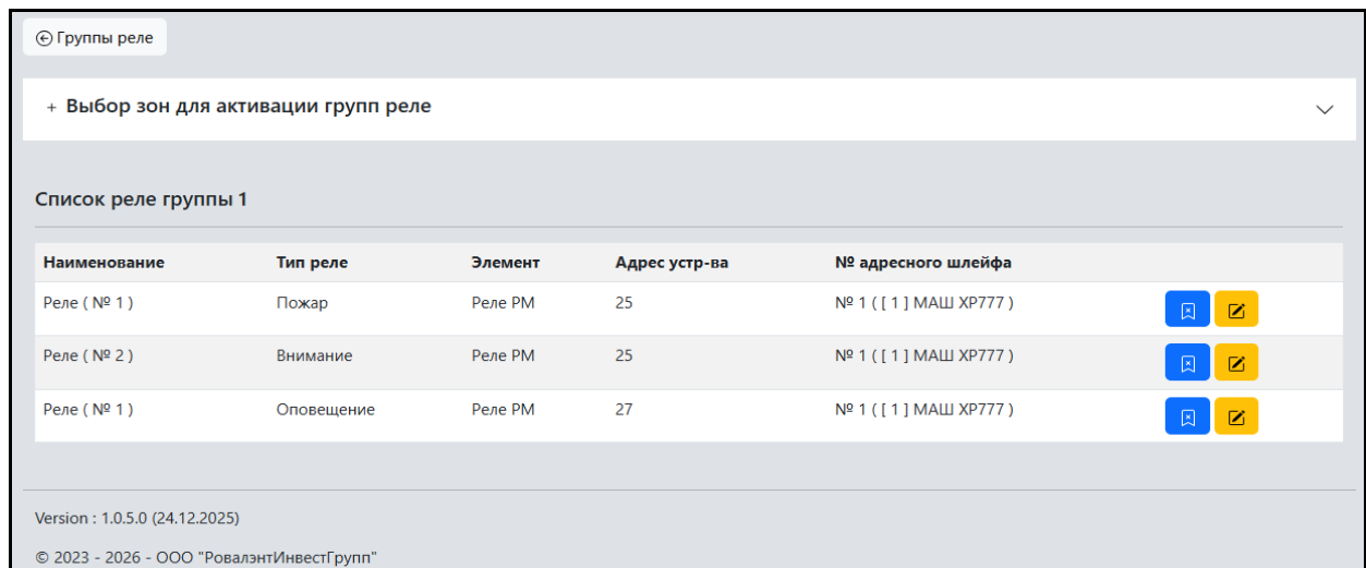
Рис. 54. Скриншот окна вкладки «Список реле группы 1»
