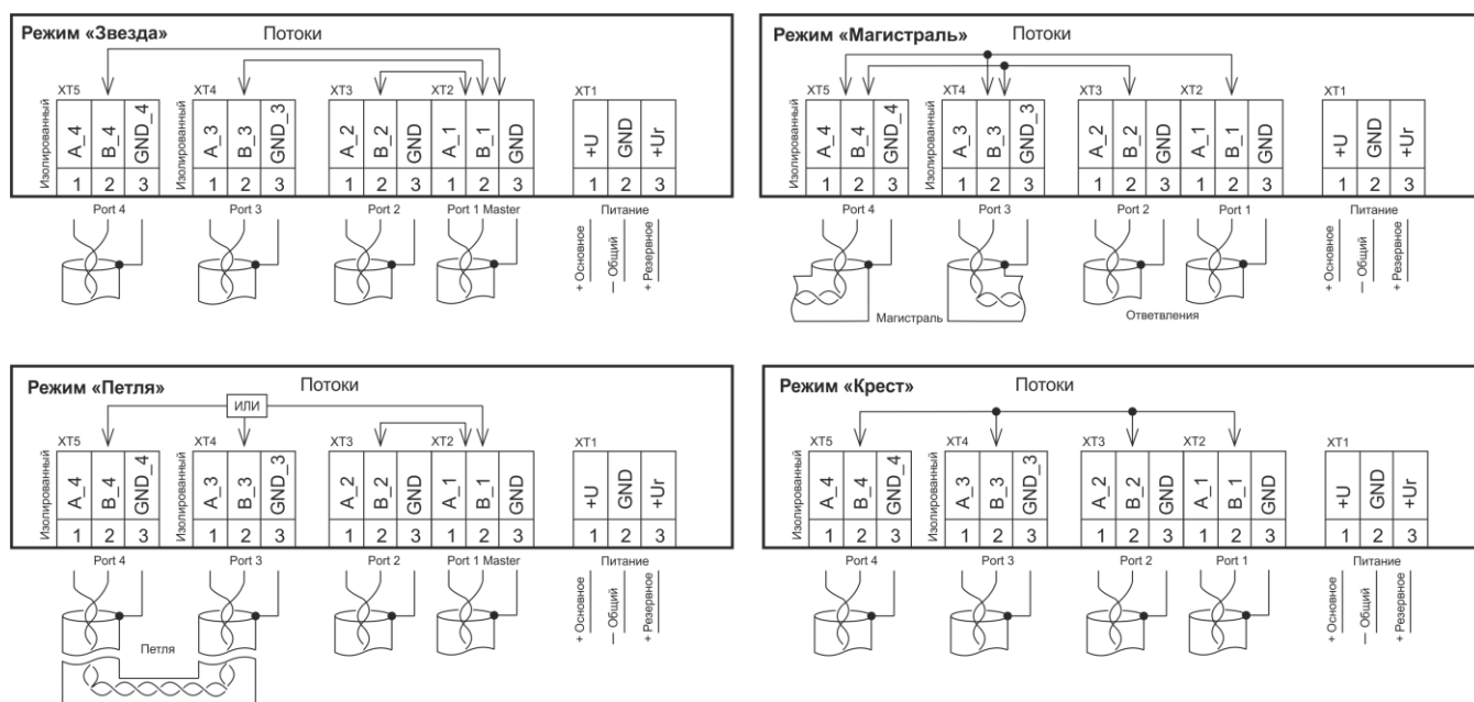
Рис. 54. Подключение P485 при различных режимах его работы
