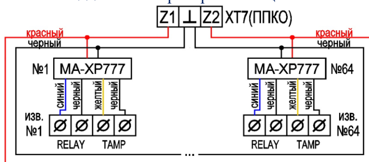
Рис. 56. Схема подключения МА-ХР777
