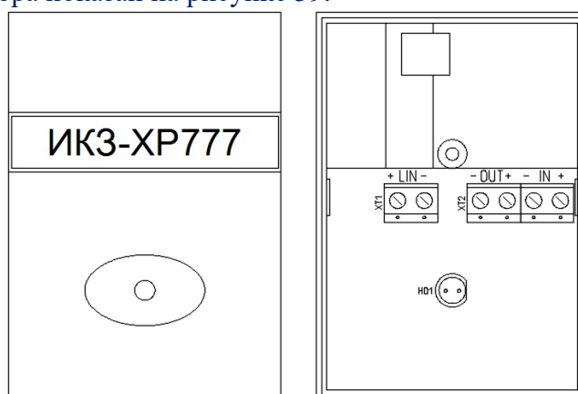
Рис. 59. Внешний вид лицевой панели и платы ИКЗ-ХР777
