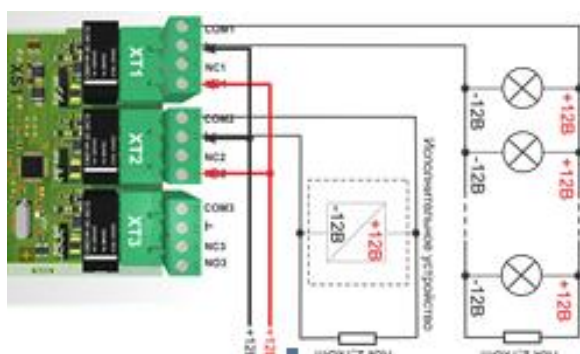
Рис. 6. Внешний вид и обозначение элементов РМ-А24/3
