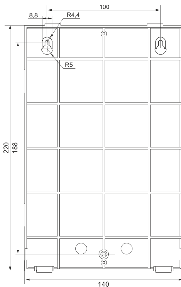
Рис. 64. Установочный чертеж ПИУ-А24Б(О)
