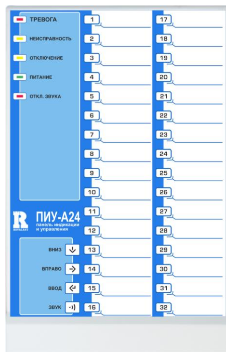
Рис. 47. Внешний вид лицевой панели ПИУ-А24Б(О)
