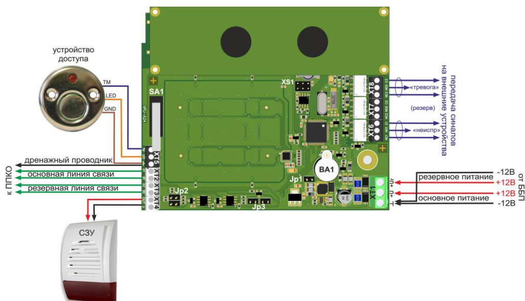
Рис. 8. Внешний вид и схема подключения платы ВПУ-А24/700(О)
