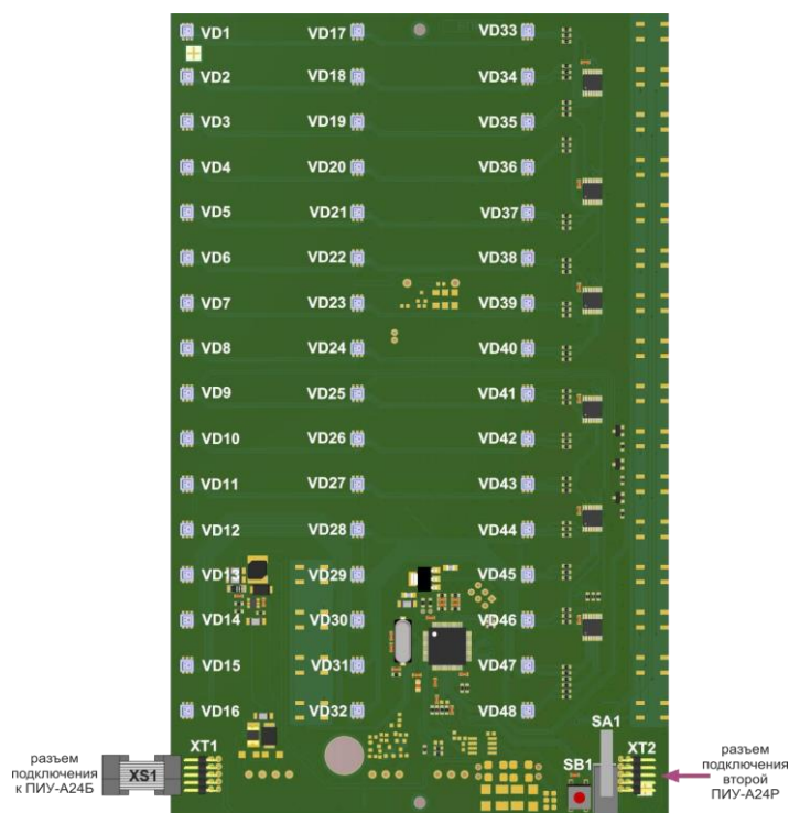
Рис. 51. Внешний вид платы ПИУ-A24P(O), обозначение элементов и схема подключения Назначение элементов и контактов на плате ПИУ-A24P(O) приведено в таблице 32.
