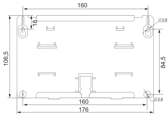
Рис. 63. Установочный чертеж основания корпуса Р485
