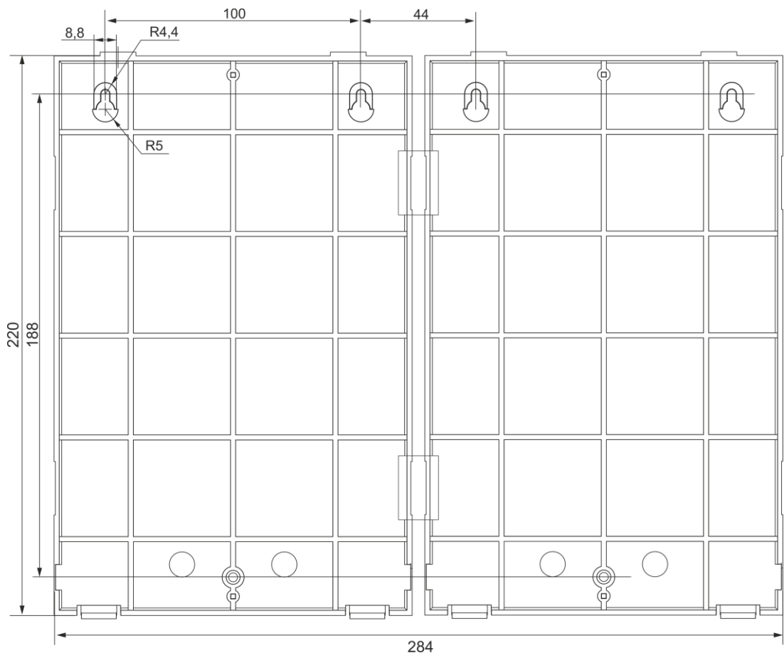
Рис. 65. Установочный чертеж ПИУ-А24Б(О) с одной подключенной ПИУ-А24Р(О)
