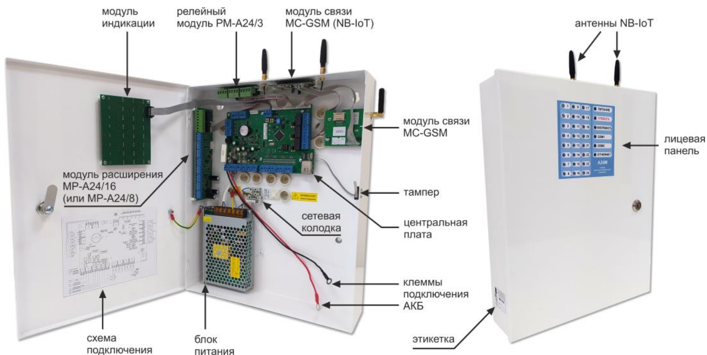
Рис. 1. Внешний вид и состав ППКО
