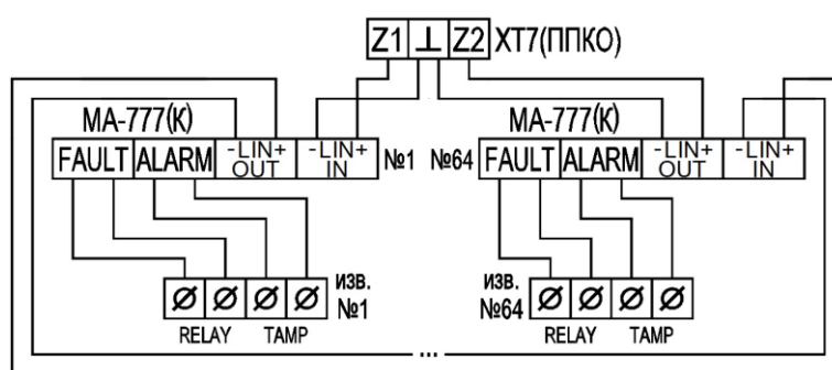
Рис. 58. Схема подключения МА-ХР777(К)
