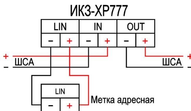
Рис. 60. Схема подключения изолятора
