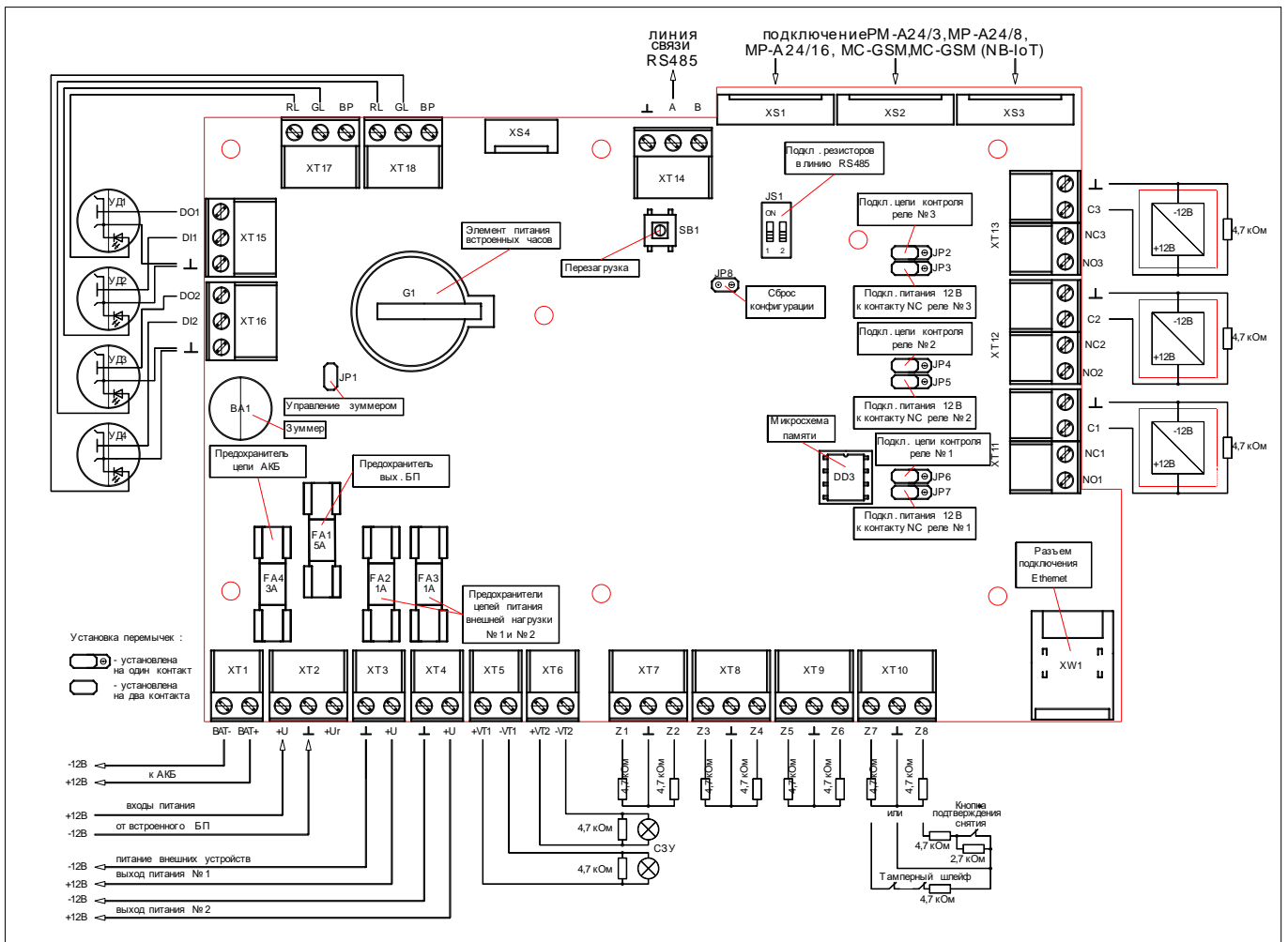
Рис. 2. Схема внешних подключений центральной платы ППКО А24/8М
