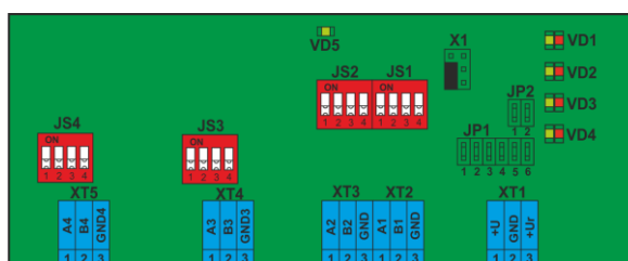
Рис. 53. Внешний вид платы P485
