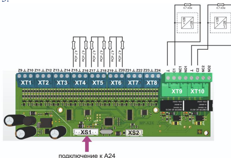
Рис. 5. Внешний вид и схема подключения МР-А24/16
