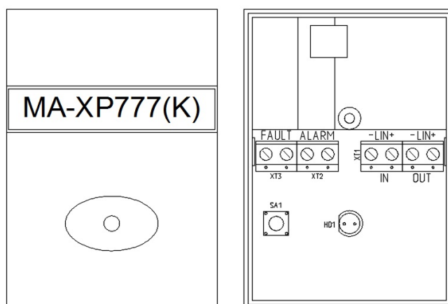
Рис. 57. Внешний вид лицевой панели с накладкой и платы МА-ХР777(К)
