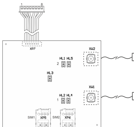
Рис. 4.1. Внешний вид модуля связи MC-GSM (NB-IoT)
