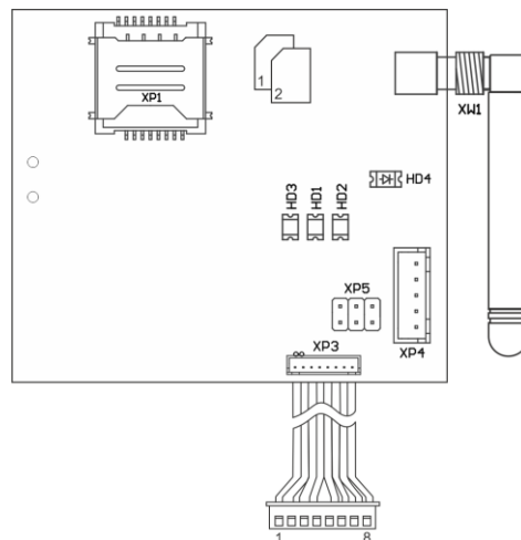
Рис. 4. Внешний вид MC-GSM
