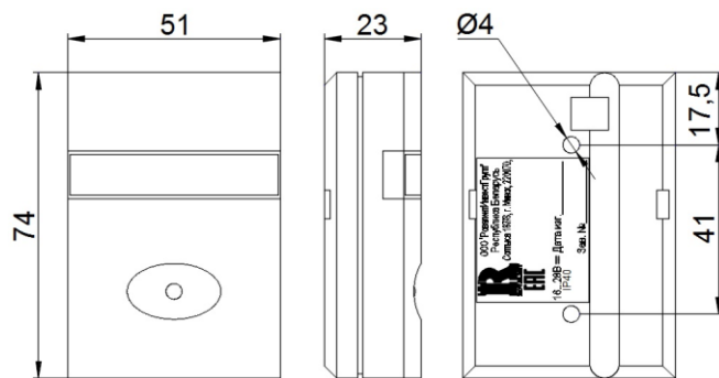
Рис. 66 Установочный чертеж МА-ХР777(К) и ИКЗ-ХР777
