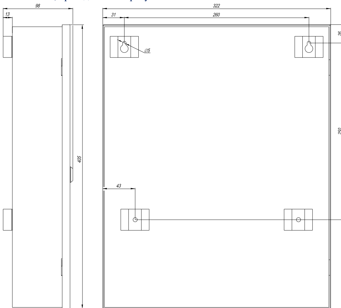
Рис. 61. Установочный чертеж основания корпуса ППКО серии «A24M»
