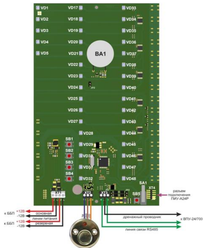
Рис. 48. Внешний вид и подключение платы ПИУ-A24B(O)
