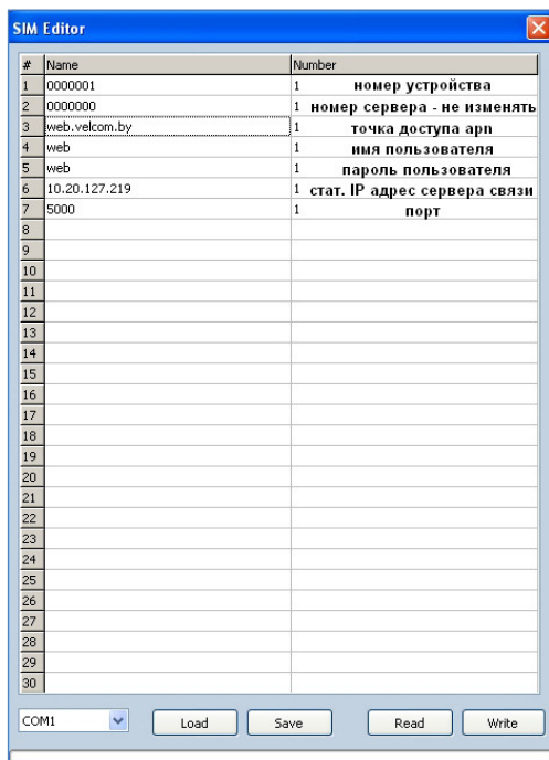
Рис. 3. Скриншот окна программатора «Sim Editor» и пример программирования SIM-карты для работы в составе СПИ «Неман»
