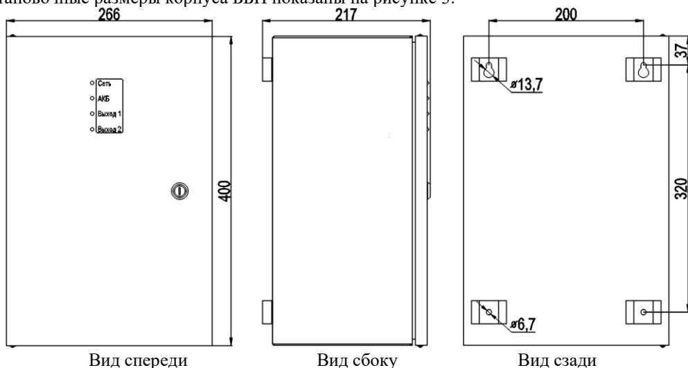
Рис. 3 Внешний вид, габаритные и установочные размеры корпуса ББП
