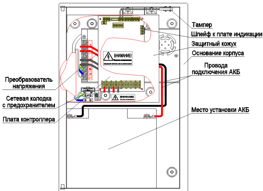
Рис. 1 Внешний вид и расположение конструктивных элементов БПП (при снятом защитном кожухе и открытой лицевой панелию)
