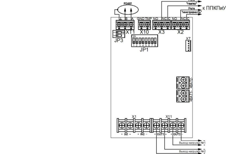
Рис. 2 Внешний вид платы контроллера и схема внешних подключений ББП
