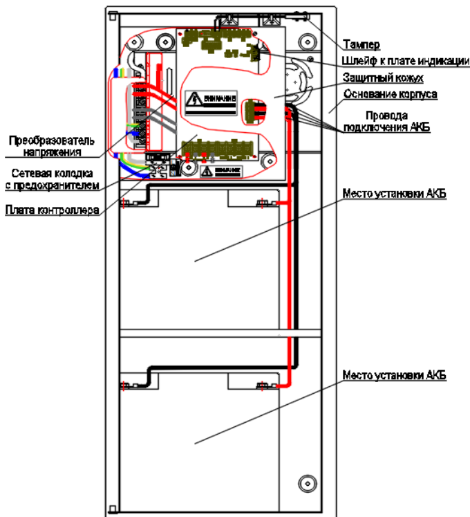
Рис. 1 Внешний вид и расположение конструктивных элементов БПП (при снятом защитном кожухе и открытой лицевой панелью)
