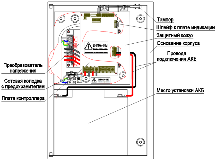
Рис. 1 Внешний вид и расположение конструктивных элементов БПП (при снятом защитном кожухе и открытой лицевой панели)
