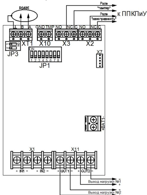
Рис. 2 Внешний вид платы контроллера и схема внешних подключений БПП
