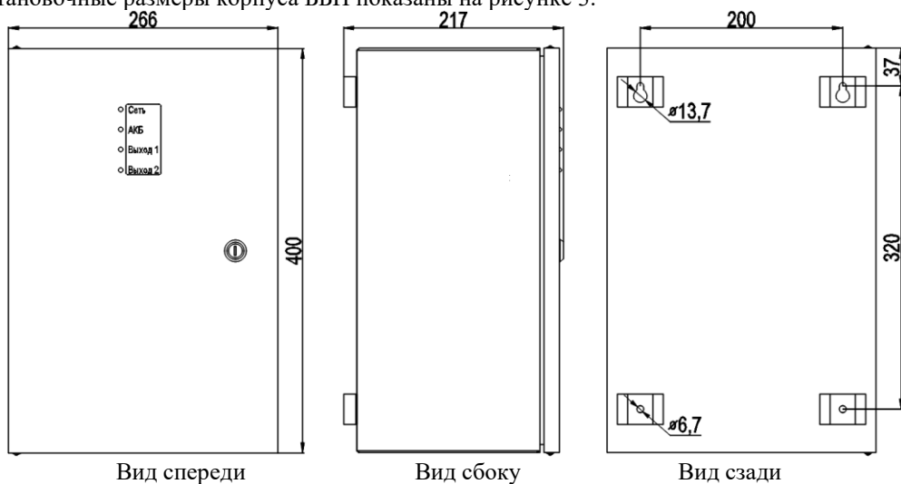
Рис. 3 Внешний вид, габаритные и установочные размеры корпуса ББП
