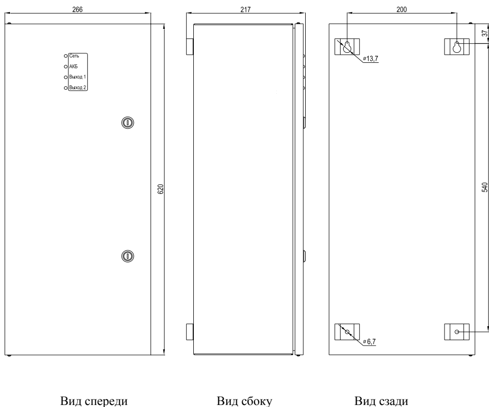
Рис. 3 Внешний вид, габаритные и установочные размеры корпуса ББП
