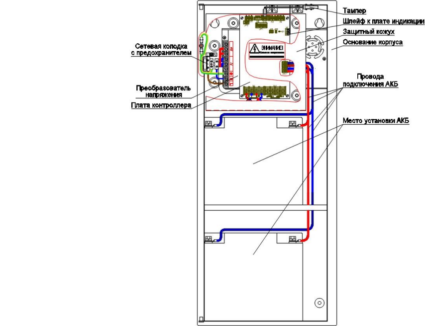
Рис. 1 Внешний вид и расположение конструктивных элементов ББП (при снятом защитном кожухе)
