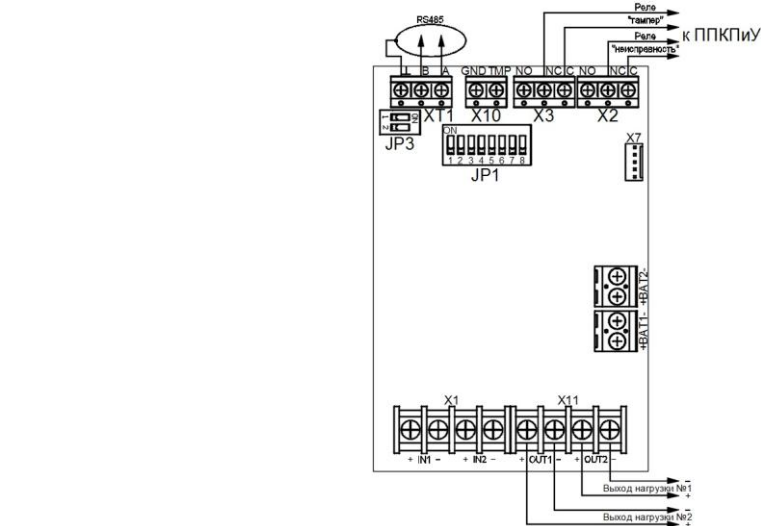
Рис. 2 Внешний вид платы контроллера и схема внешних подключений ББП
