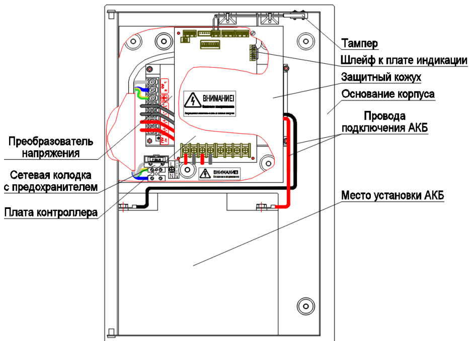
Рис. 1 Внешний вид и расположение конструктивных элементов БПП (при снятом защитном кожухе и открытой лицевой панелью)
