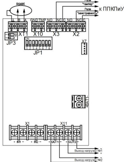
Рис. 2 Внешний вид платы контроллера и схема внешних подключений БП
