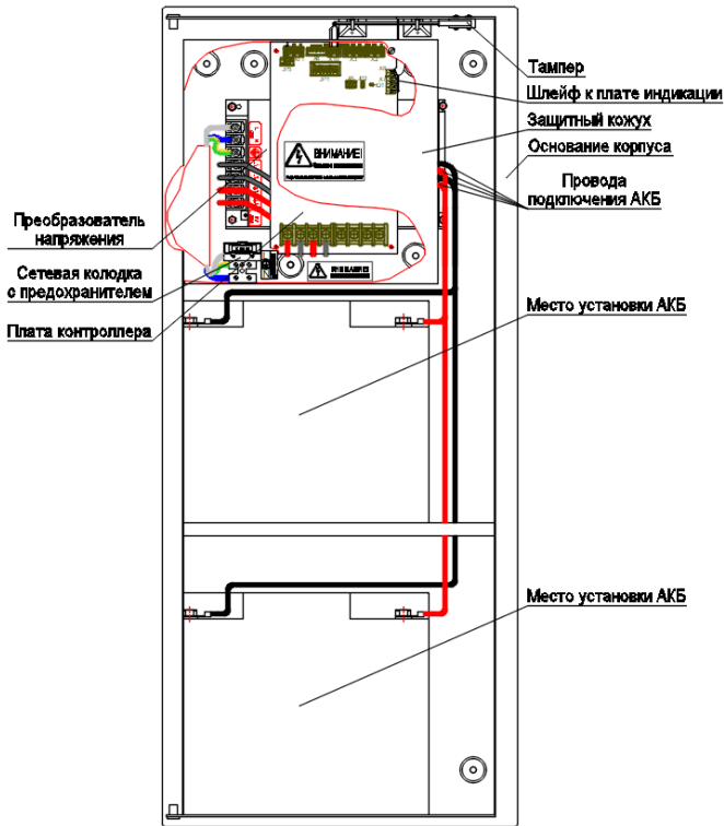
Рис. 1 Внешний вид и расположение конструктивных элементов БП (при снятом защитном кожухе и открытой лицевой панели)
