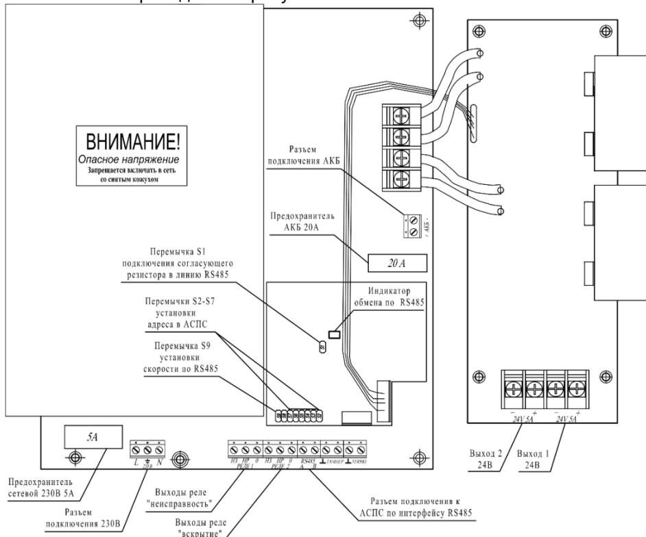
Рис. 1. Расположение контактных колодок, предохранителей, установочных элементов ББП
