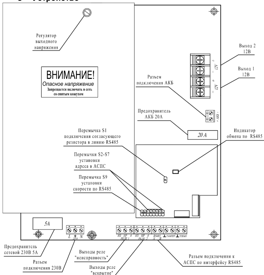
Рис. 1. Расположение контактных колодок, предохранителей, установочных элементов ББП
