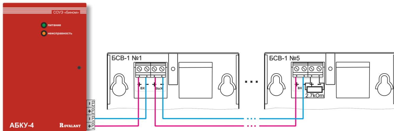
Рисунок 50. Схема подключения БСВ-1
