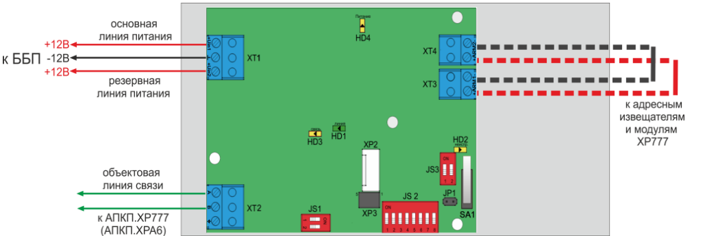
Рис. 1. Внешний вид платы модуля и схема подключений
