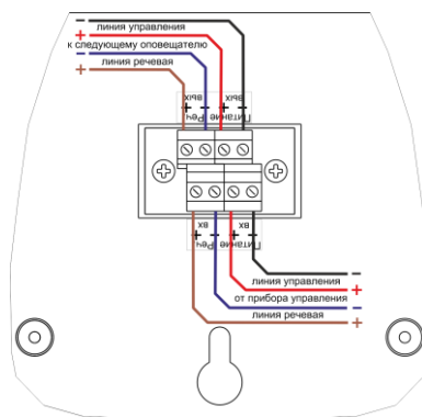
Рис.2 Схема подключения оповещателя
