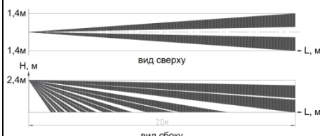
Рис. 3 Вид зоны обнаружения извещателя по ИК-каналу
