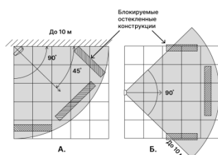
Рис. 3 Вид зоны обнаружения извещателя по ИК-каналу
