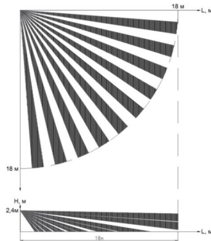
Рис. 3. Вид зоны обнаружения извещателя по ИК-каналу
