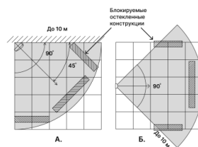
Рис. 4. Вид диаграммы направленности по АК-каналу (в горизонтальной плоскости)
