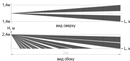
Рис. 3. Вид зоны обнаружения извещателя
