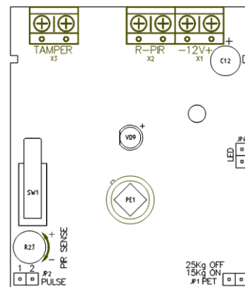
Рис. 2. Внешний вид платы извещателя
