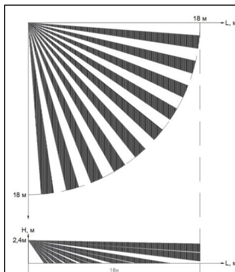
Рис. 3. Вид зоны обнаружения извещателя
