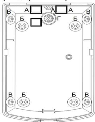
Рис. 4. Внешний вид внутренней стороны основания корпуса извещателя
