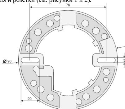
Рис. 2. Установочный эскиз розетки
