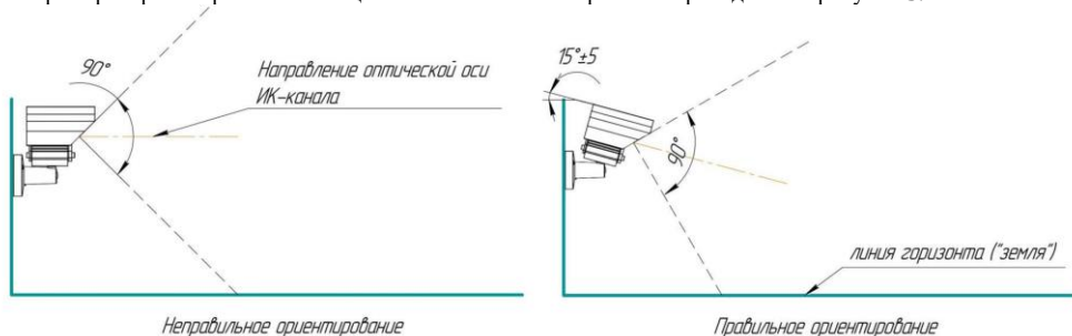
Рис. 3 Пример установки извещателя
