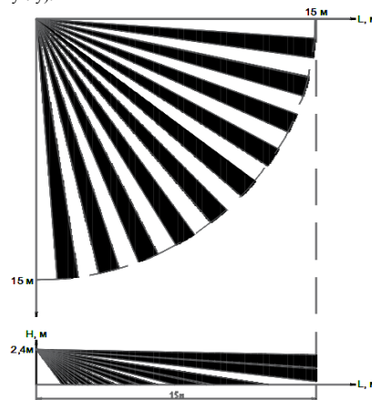
Рис. 3. Вид зоны обнаружения извещателя
