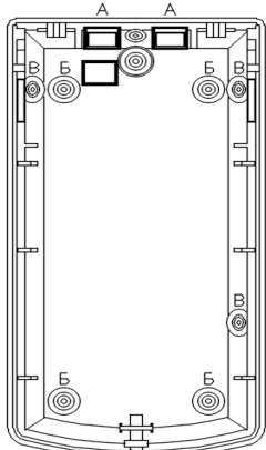
Рис. 4. Внешний вид внутренней стороны основания корпуса извещателя
