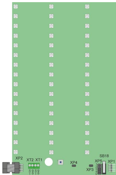
Рис.2. Внешний вид платы ВПИУ-люкс (расширение до 8)
